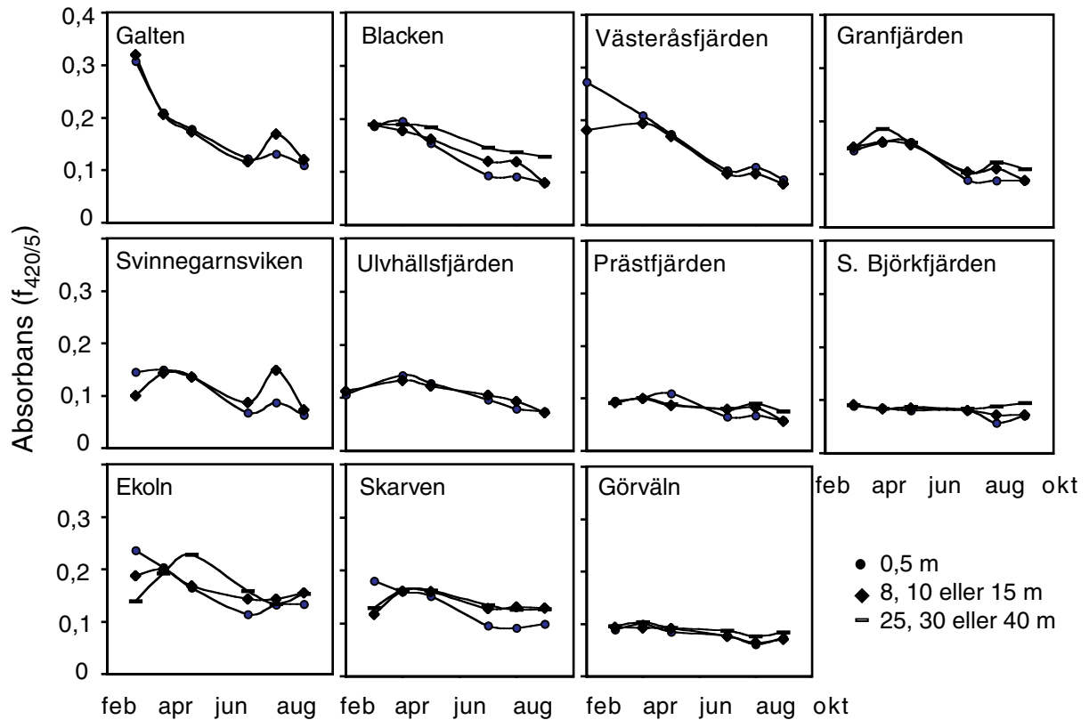
Figur 10. Vattenfärg, mätt som absorbans på filtrerat vatten (0,45 \mu\text{m} membranfilter) i 5 cm kyvett vid 420 nm våglängd ( f_{420/5} ) i Mälarens fjärdar på olika nivåer under provtagningsåret 2002.
