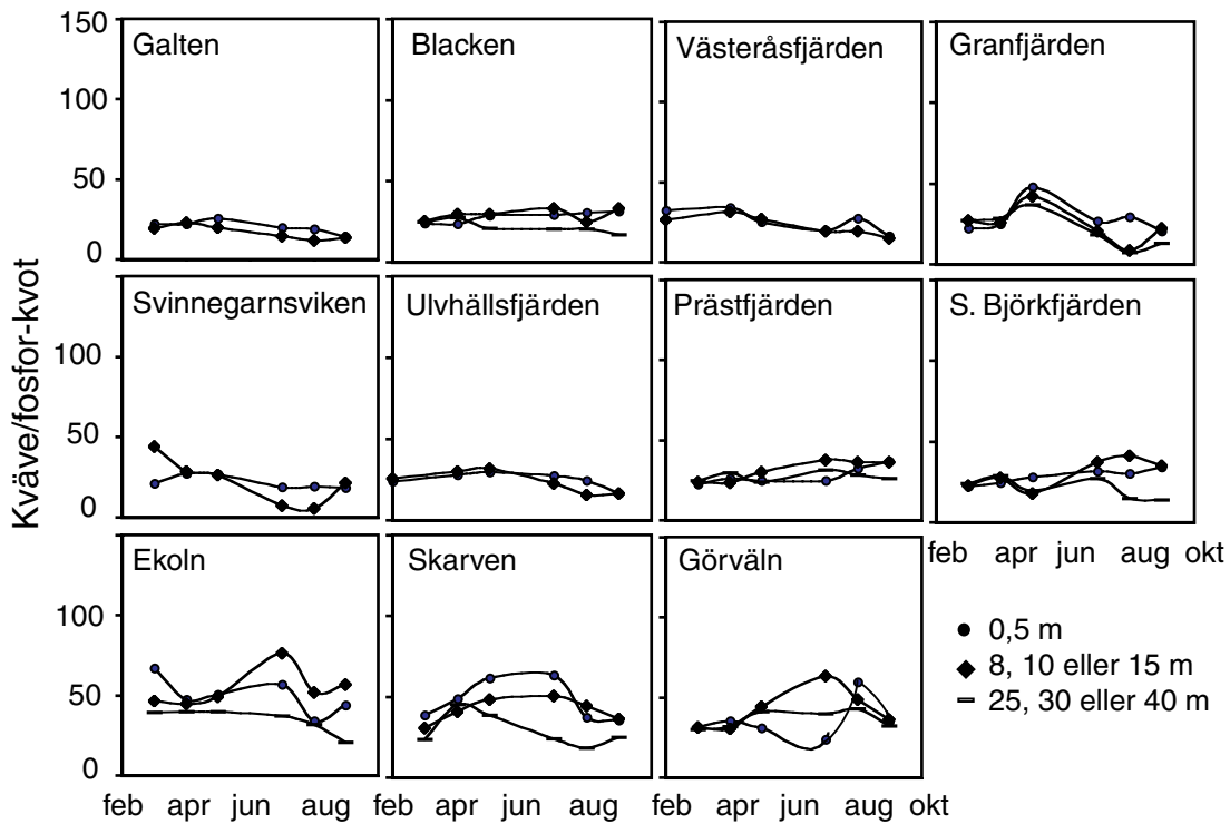
Figur 18. Totalkväve/totalfosforkvoten i Mälarens fjärdar på olika nivåer under provtagningsåret 2002.
