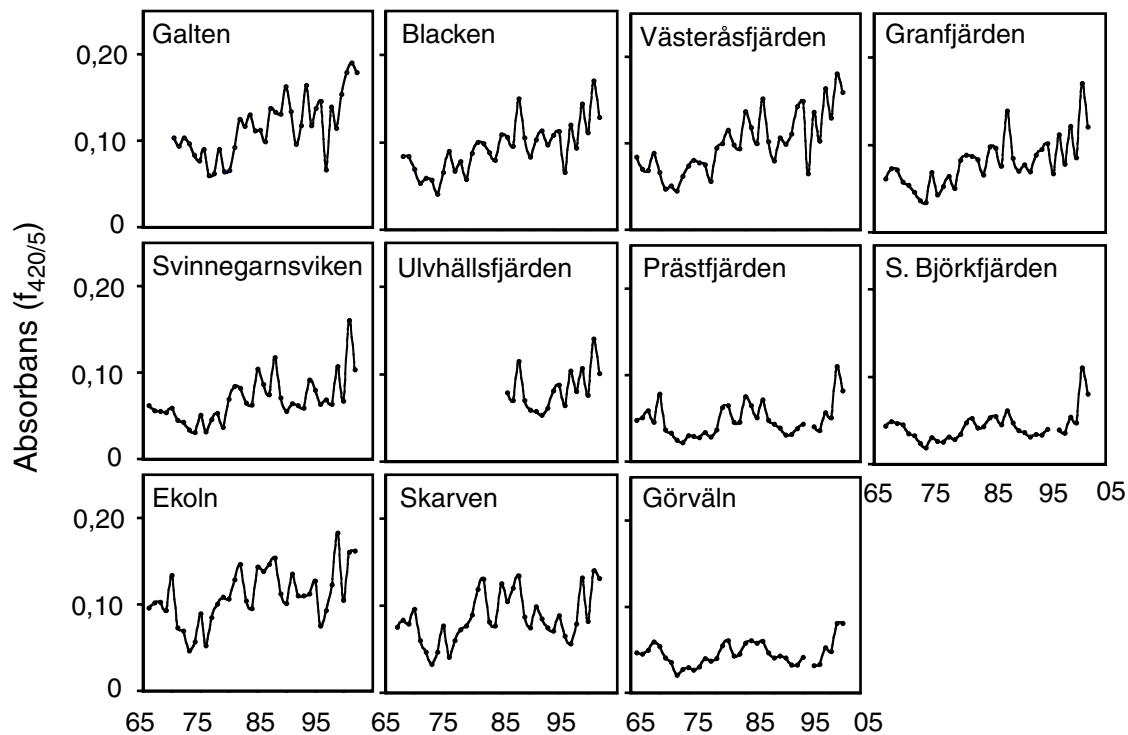
Figur 20. Vattenfärg (medel från februari/mars, maj, juli och september), mätt som absorbans på filtrerat vatten (0,45 \mu\text{m} membranfilter) i 5 cm kyvett vid 420 nm våglängd ( f_{420/5} ) i Mälarens ytvatten (0,5 m) de senaste 38 åren.
