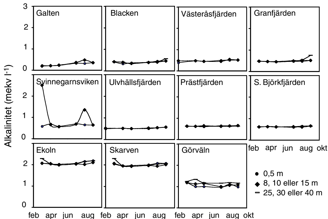
Figur 11. Alkalinitet i Mälarens fjärdar på olika nivåer under provtagningsåret 2002.
